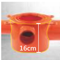
切邊設計
