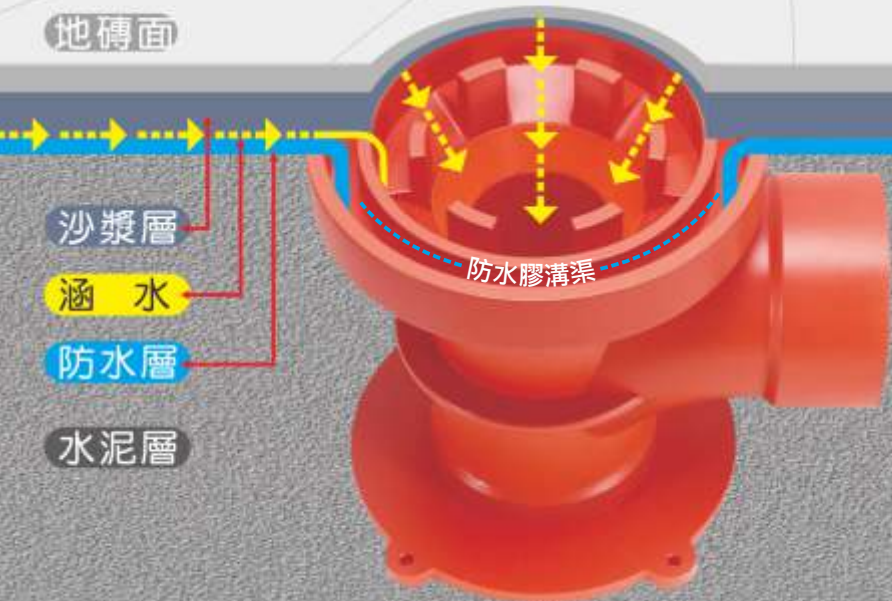
BA129-D 暗排水防臭順水T 口徑：3"x2½"x2" 材質：PVC
