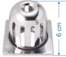
PD739 PD739A (附網) 不鏽鋼高腳落水頭 尺寸：9.3x9.3x6cm 口徑：1½", 2", 3"
