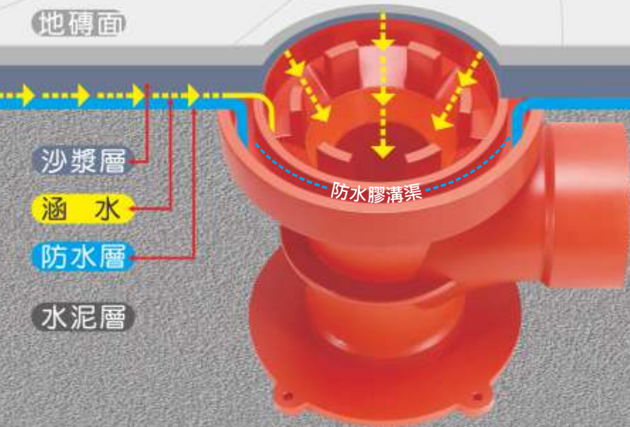
BA129-D 暗排水防臭順水 T 口徑：3"x2 1/2"x2" 材質：PVC
